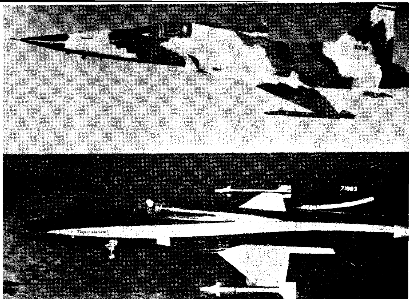
Arriba un Northrop F-5E Tiger-II. Abajo el F-5G Tigershark que es un desarrollo avanzado del anterior con elementos comunes y otros de nuevo diseño.
